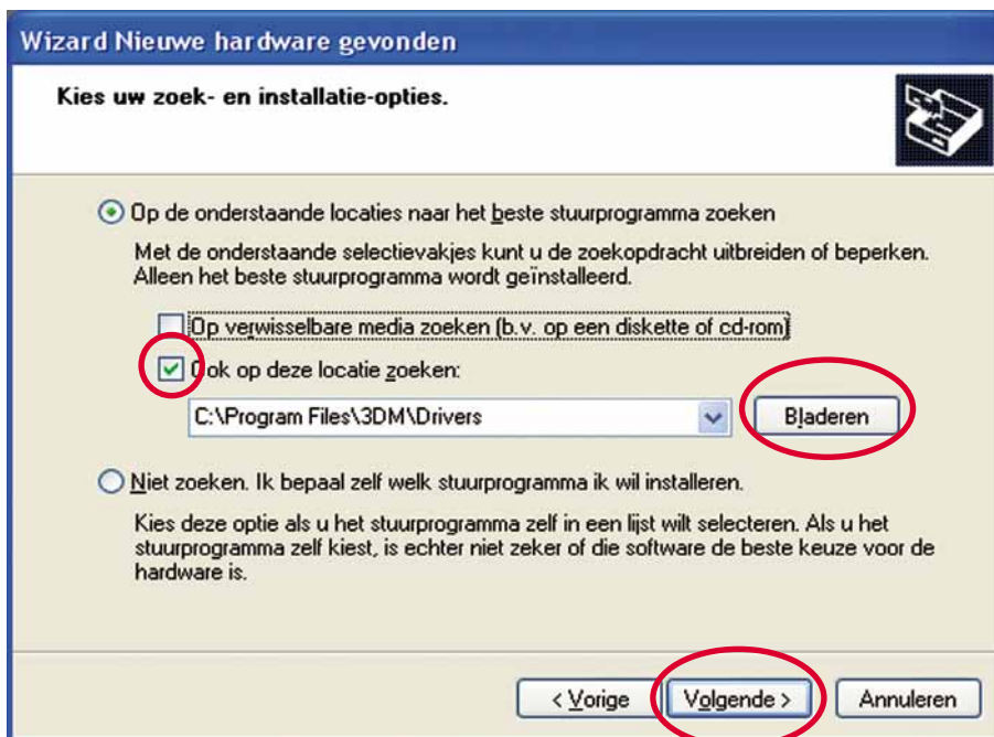
Figuur 11: Installatie responsbox Windows XP en Vista.
